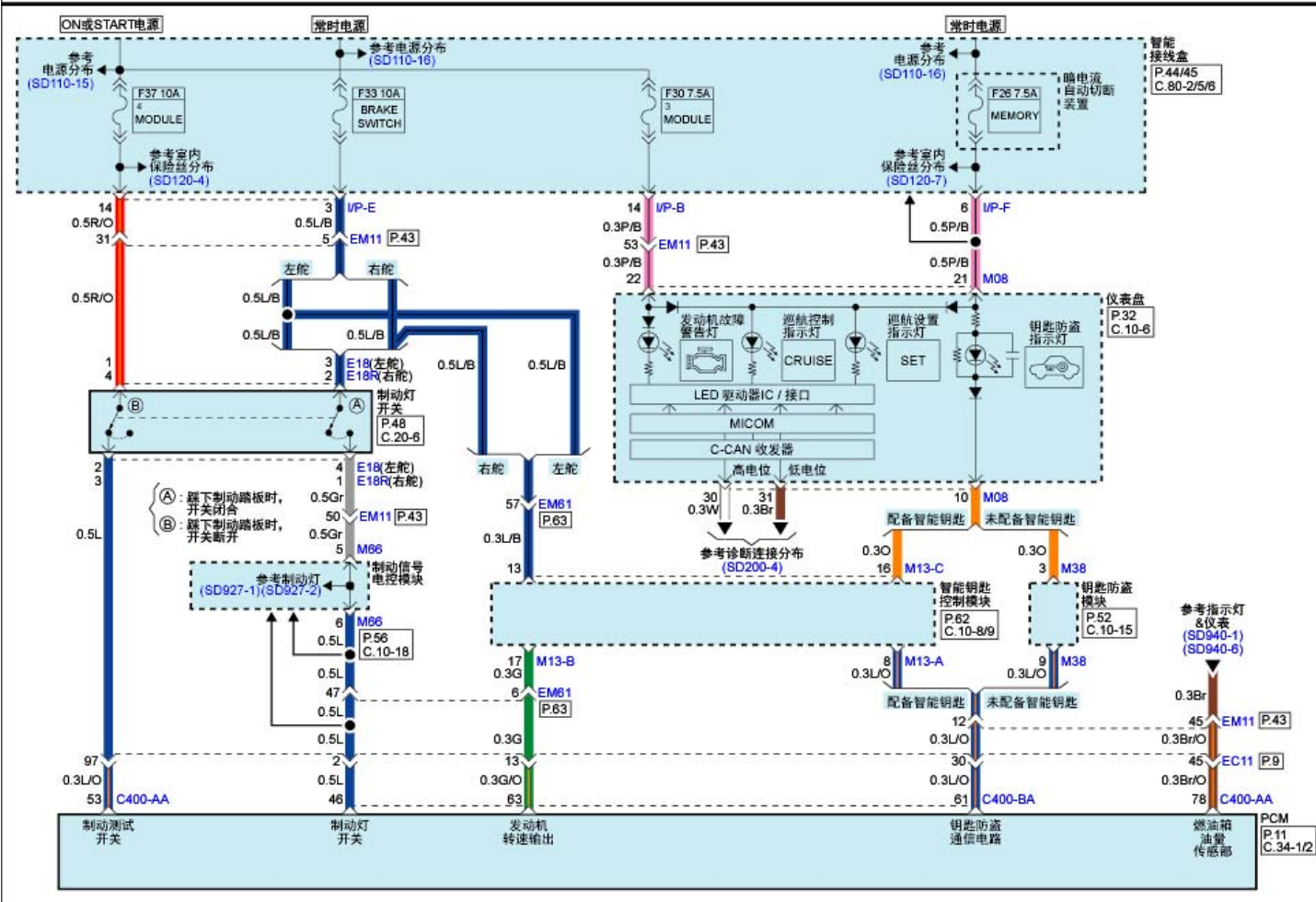
发动机控制系统(G4FJ: GAMMA 1.6L T-GDI A/T)(7)
